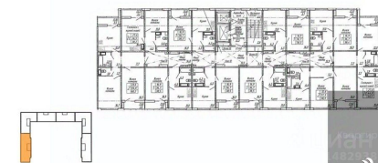
КОРПУС 7 Секция 1 План 2-16 этажей
