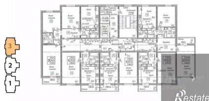
КОРПУС 46 Секция 3 План 2-17 этажей
