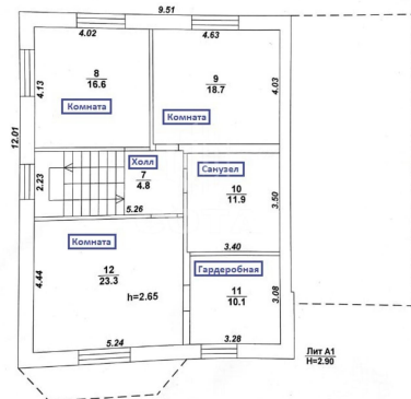
Мансарда 85,4 м 2
